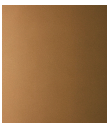
Jupiter
